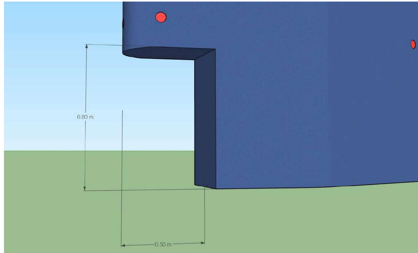
DETAIL DES ENCOCHES BASSES
